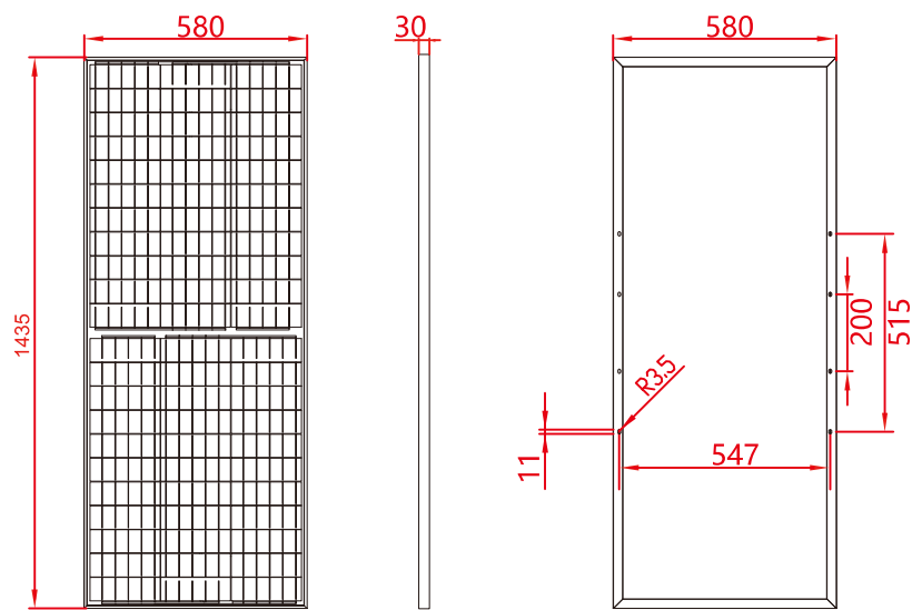
150W/18V
